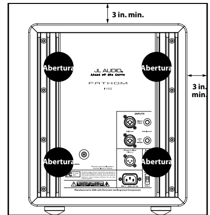
Vista trasera de la instalación del gabinete:
