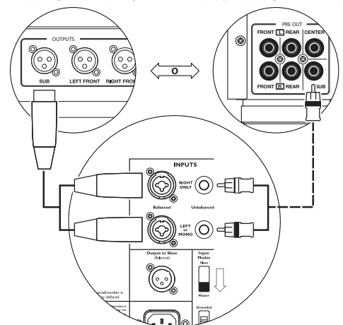
PANEL DE CONTROL POSTERIOR DE UN SUBWOOFER FATHOM (MAESTRO)
