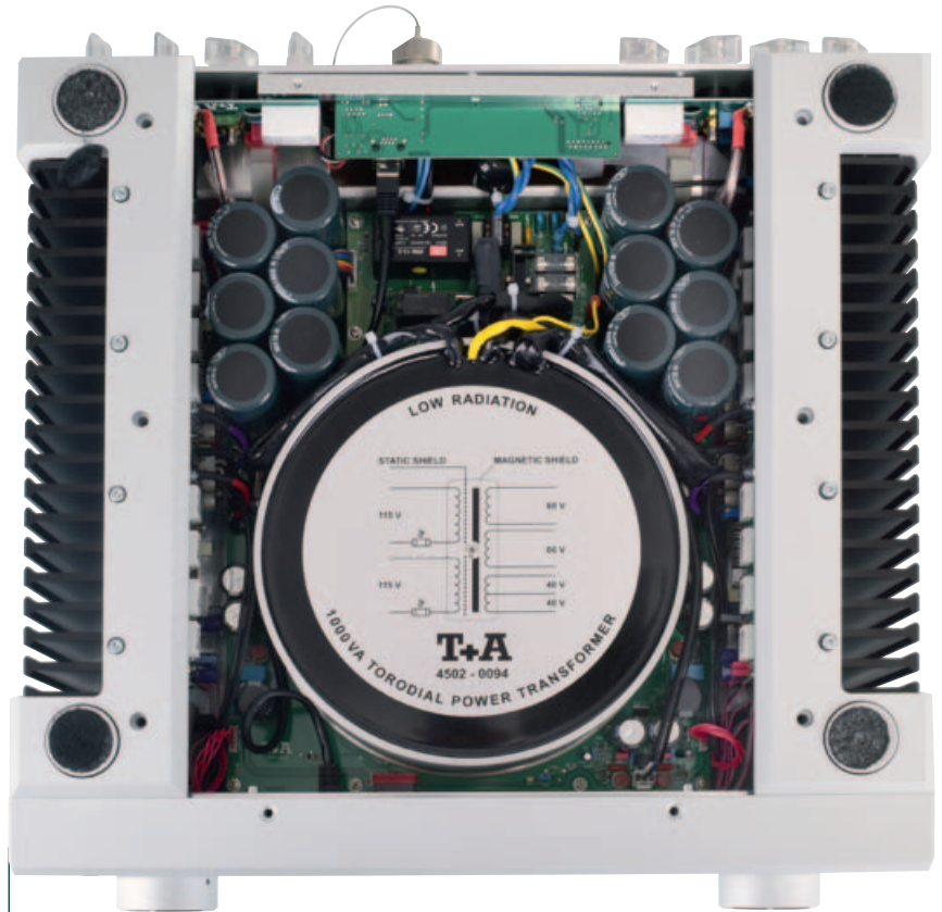
GEBEN, WAS GEBRAUCHT WIRD: Hebt man den Deckel des PA 3100 HV ab, fällt der gewaltige Ringkerntransformator ins Auge. Gemeinsam mit den Siebkapazitäten von 120 000 Mikrofarad stellt er die Stromversorgung vieler Endstufen in den Schatten.
